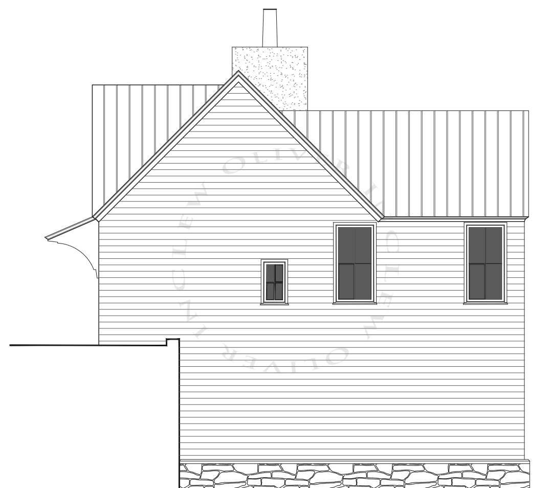
RIGHT ELEVATION
